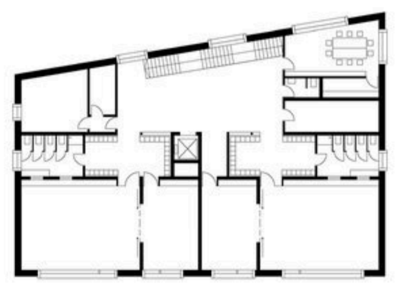
OBERGESCHOSS
