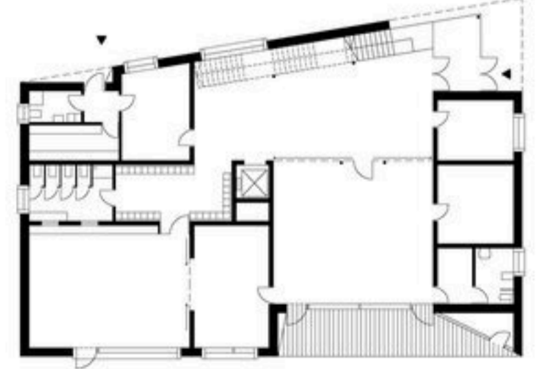
ERDGESCHOSS
