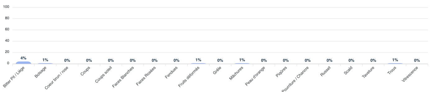
Défauts (500 fruits)
