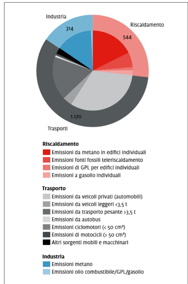
Emissioni di CO 2 equivalenti in Alto Adige da fonti fossili, dati 2019 (Settore agricolo non riportato nel diagramma). Elaborazione Eurac Research su dati APPA
