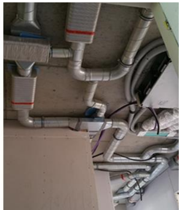
Impianti casa plurifamiliare Aurum, Ora
